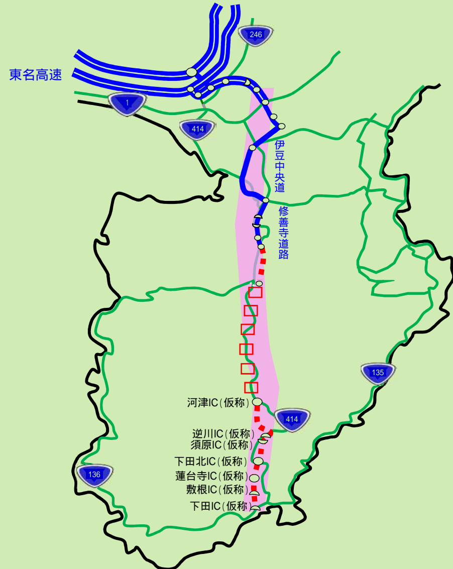
伊豆半島の広域道路ネットワーク
